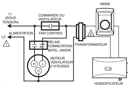
Fig. 12. Raccordement du H8908 avec asservissement du ventilateur.
