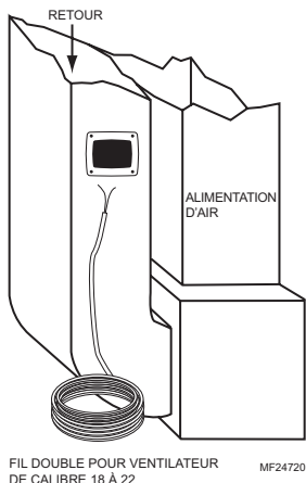
Fig. 5. Amener le fil jusqu'à l'emplacement de montage.
