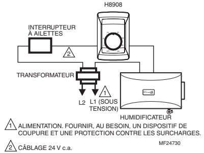
Fig. 15. Raccordement du H8908 en série avec un interrupteur à ailettes et un humidificateur.
